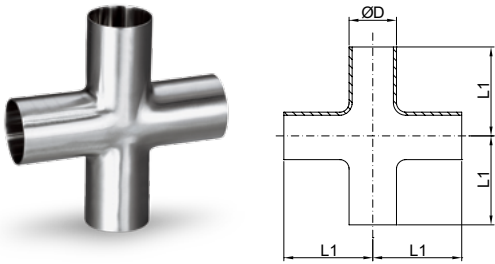
卡箍式四通 Clamped Cross
