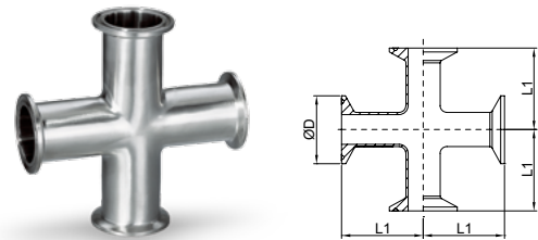
卡箍式四通 Clamped Cross
